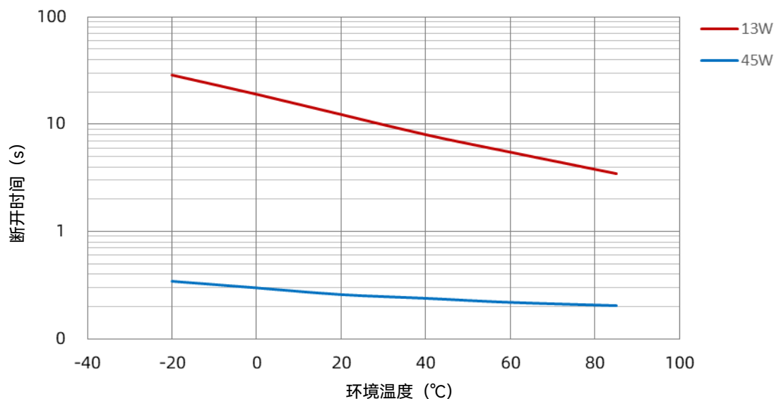
SHL 30 A 功率-温度曲线
